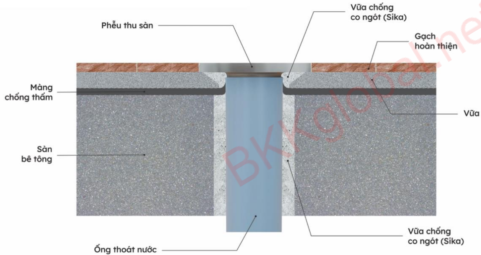
Mô hình 7 lớp kết cấu tại phễu
